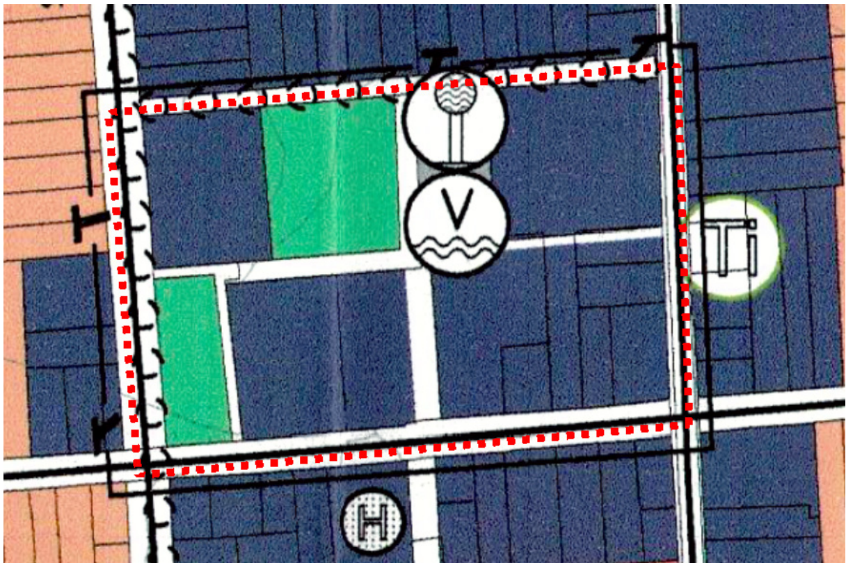
Hatályos és fenntartott településszerkezeti terv
