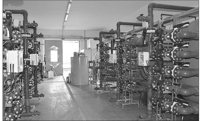
Víztisztító berendezések a József Attila utcai telephelyen Fotó: Cs. Szabó Zsuzsanna
